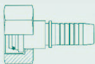
Fêmea Métrica
